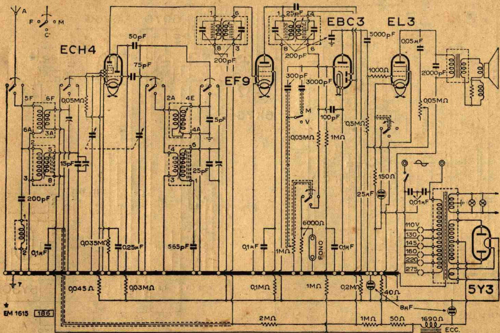
La Voce del Padrone - Columbia - Marconiphone, Mod. V.d.P. 570. (Telaio 701)
