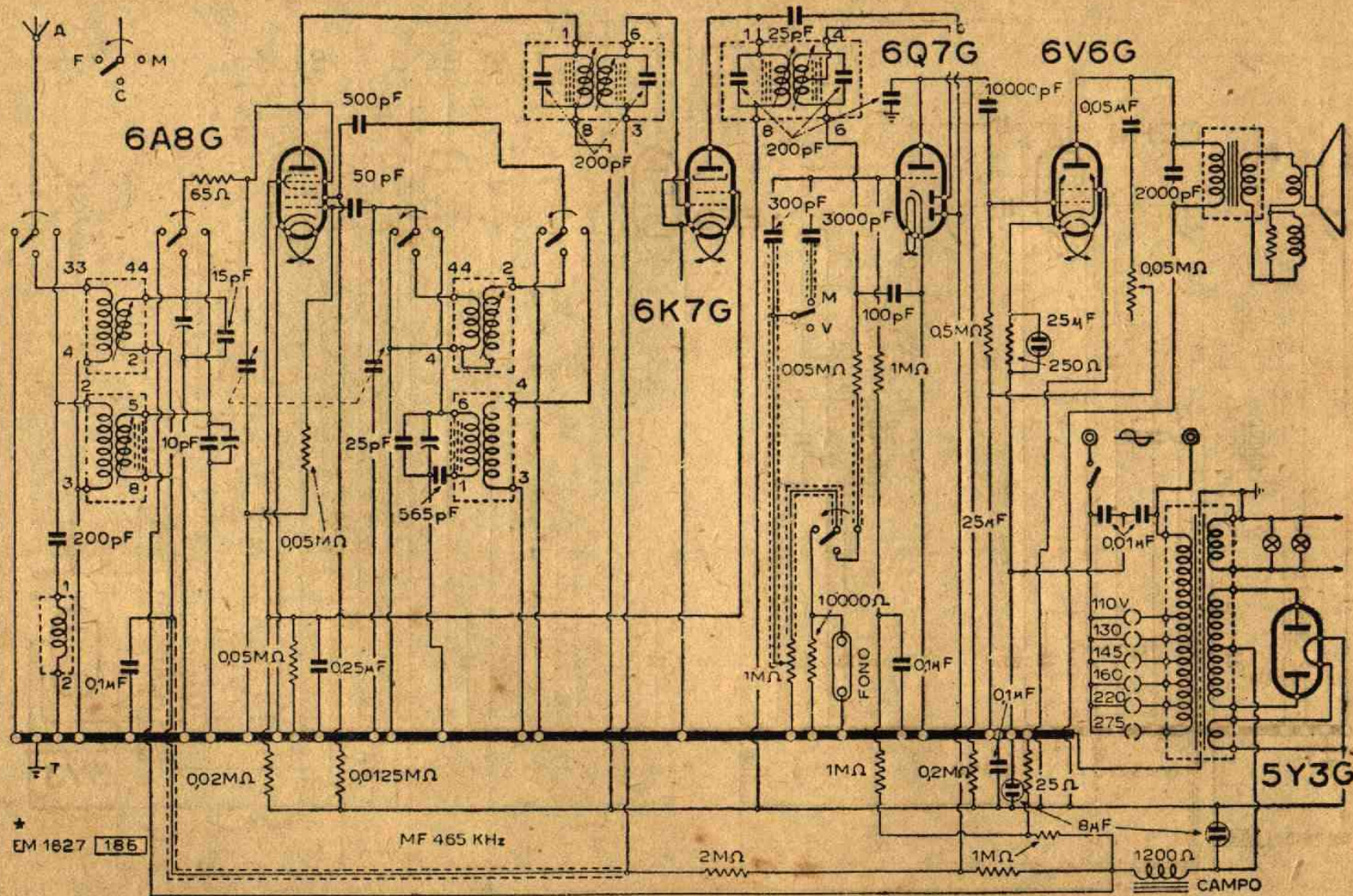
La Voce del Padrone - Columbia - Marconiphone, Mod. V. d. P. 570 A. (Telaio 70'1 A)
